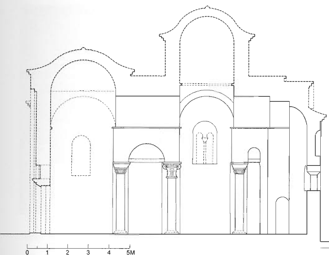
Εικ. 7. Τρίγλεια. Ναός Παντοβασιλίσσας. Τομή κατά μήκος. Αναπαράσταση (σκαρίφημα).
