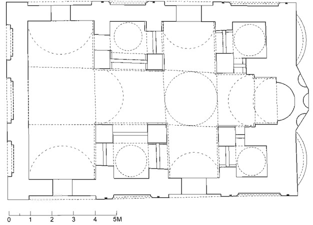
Εικ. 5. Τρίγλεια. Ναός Παντοβασιλίσσας. Κάτοψη Β. Αναπαράσταση (σκαρίφημα).
