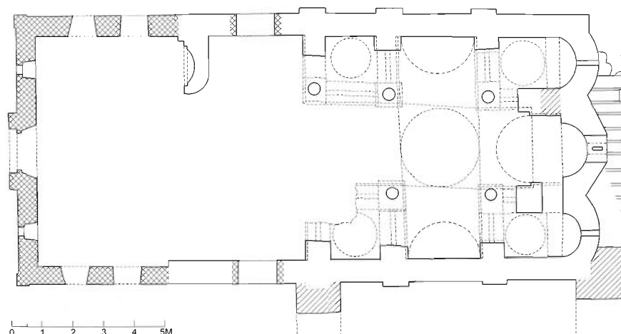
Εικ. 1. Τρίγλεια. Ναός Παντοβασιλίσσας. Κάτοψη (βάσει σχεδίων των Mango - Ševčenko, Marmara, εικ. 20 και Pekak, Zeytinbaği/Trilye, σχέδ. 6).
