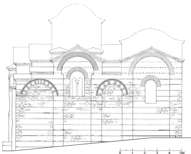
Εικ. 8. Τρίγλεια. Ναός Παντοβασιλίσσας. Βόρεια όψη. Αναπαράσταση (σκαρίφημα).
