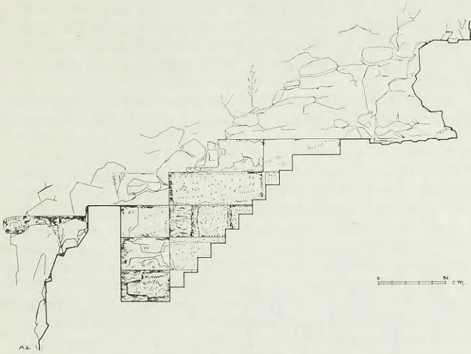
Εικ. 30. Τομή της κλίμακος της κλεψύδρας.
