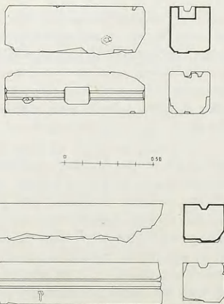
Εἰκ. 28. Ὑποδοχαὶ θωρακείων τοῦ ναοῦ.
