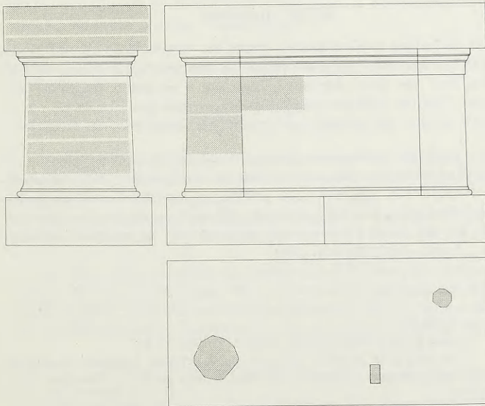
Εἰκ. 43. Τὸ βάθρον τοῦ ἀγάλματος τοῦ Ἰσαυρικοῦ.
