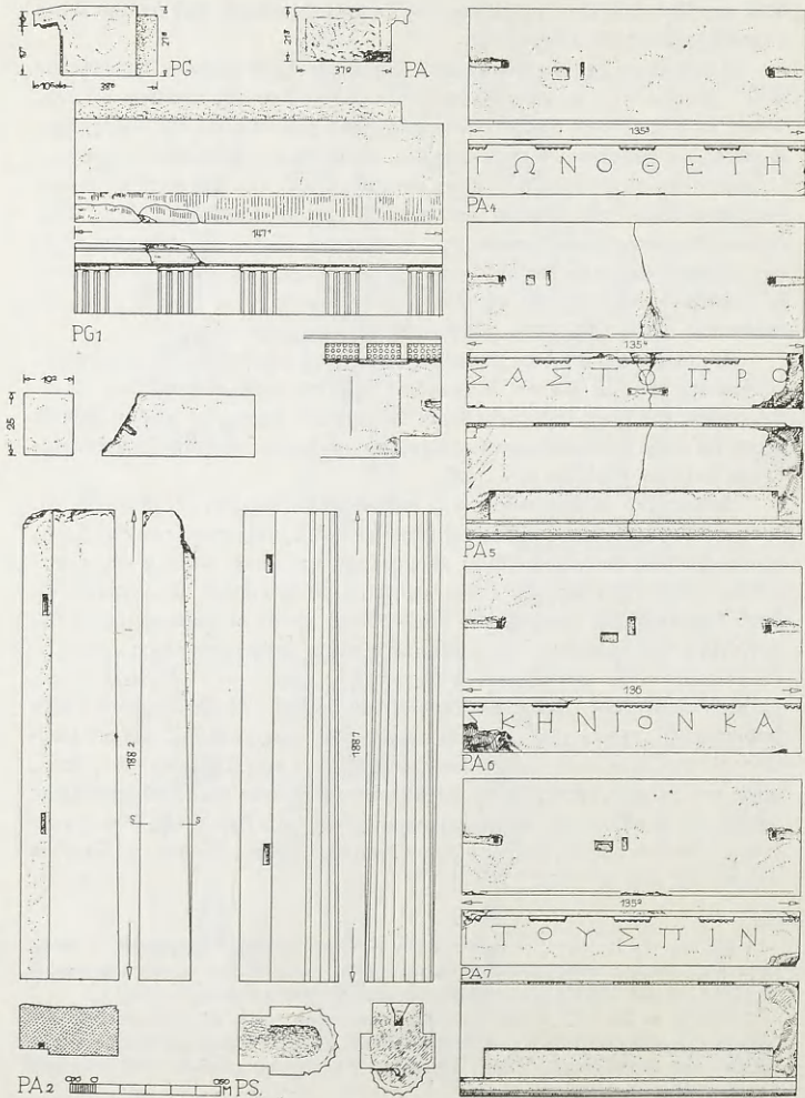
Εικ. 13. Ἐπιστύλια, τρίγλυφα καὶ γείσα προσκηνίου. Ὅψεις καὶ κάτωτις τῶν ἡμικίονων τοῦ θεάτρου κατὰ Fiechter.
