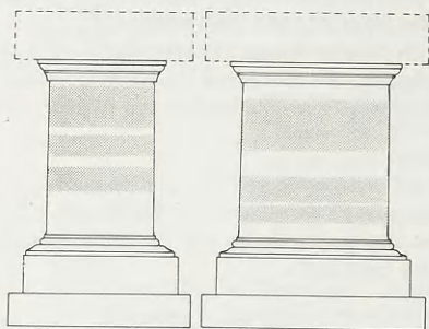
Εἰκ. 42. Τὸ βάθρον τοῦ ἀγάλματος τοῦ Μεγακλείδου.
