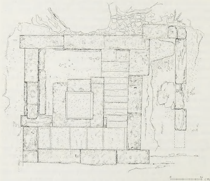
Εἰκ. 29. Κάτοπις τῆς κλεψύδρας τῆς δεξιᾶς ὄχτης τοῦ Ἱεροῦ.
