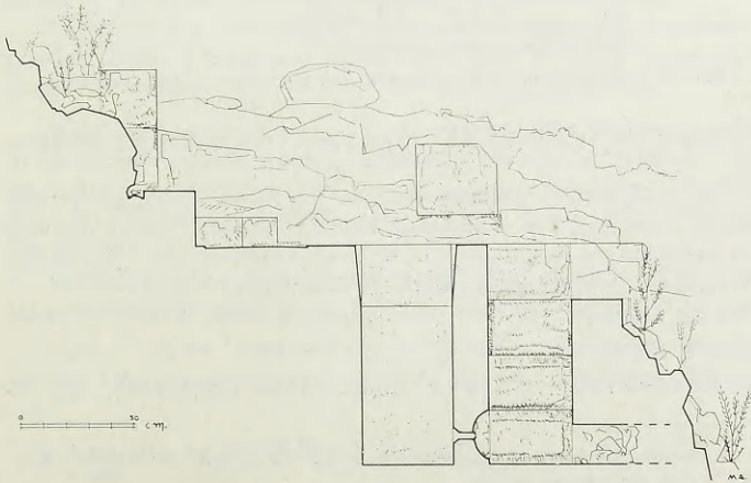
Εικ. 31. Τομή της δεξαμενής της κλεψύδρας.
