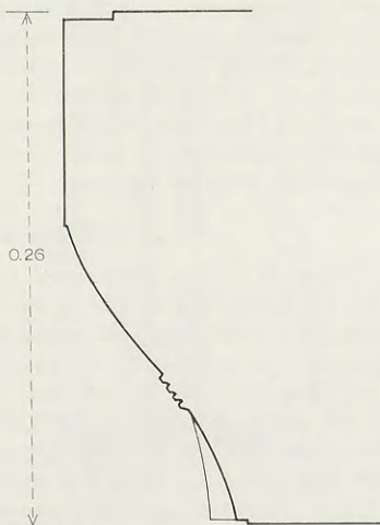
Εἰκ. 10. Τομὴ δωρικοῦ κιονοκράνου τῆς στοᾶς.
