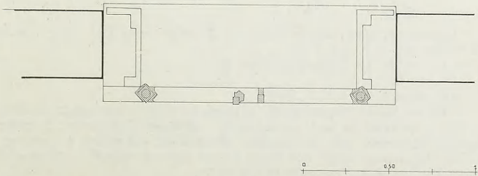
Εικ. 18. Τὸ κατόφλιον τοῦ μικροῦ ναοῦ.
