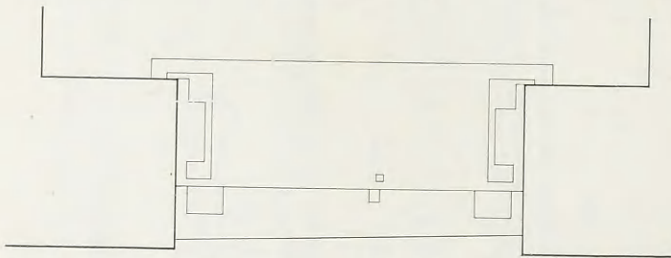
Εἰκ. 22. Τὸ δυτικὸν κατώφλιον τοῦ ναοῦ.
