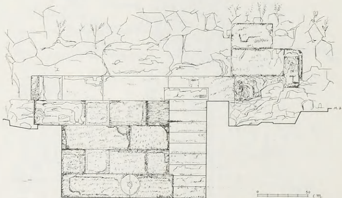
Εἰκ. 32. Ὅψεις τοῦ τοίχου τῆς δεξαμενῆς καὶ τῆς κλίμακος τῆς κλεψύδρας.
