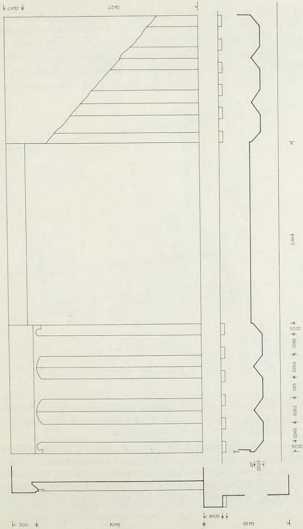
Εικόνα 7. Τριγώνων τής στούς.
