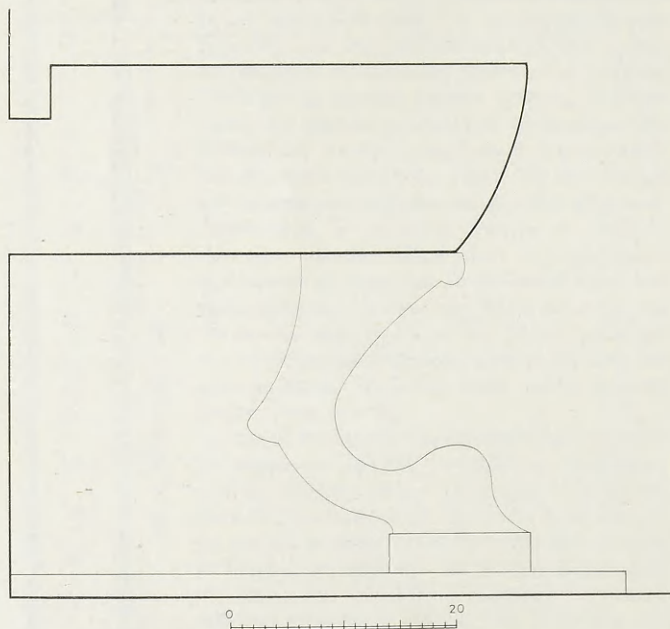
Εἰκ. 6. Τομὴ θρανίου τῆς στοᾶς.
