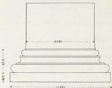
Εἰκ. 27. Ὅνις τῆς βάσεως τοῦ ἰωνικοῦ κίονος τοῦ ναοῦ κατὰ Βερσάκην.
