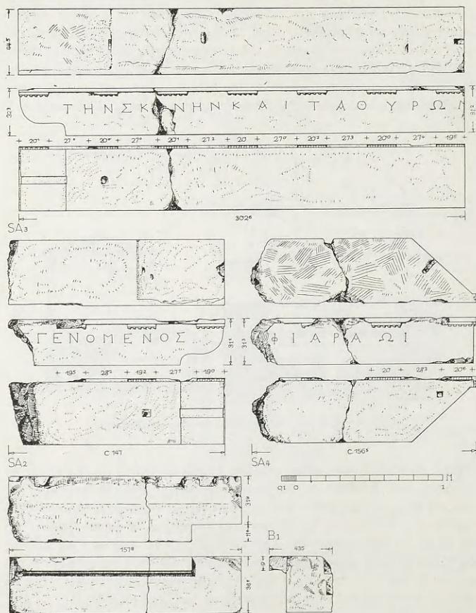
Εικ. 15. Ἐπιστόλιον τῆς σκηῆς τοῦ θεάτρου κατὰ Fiechter.
