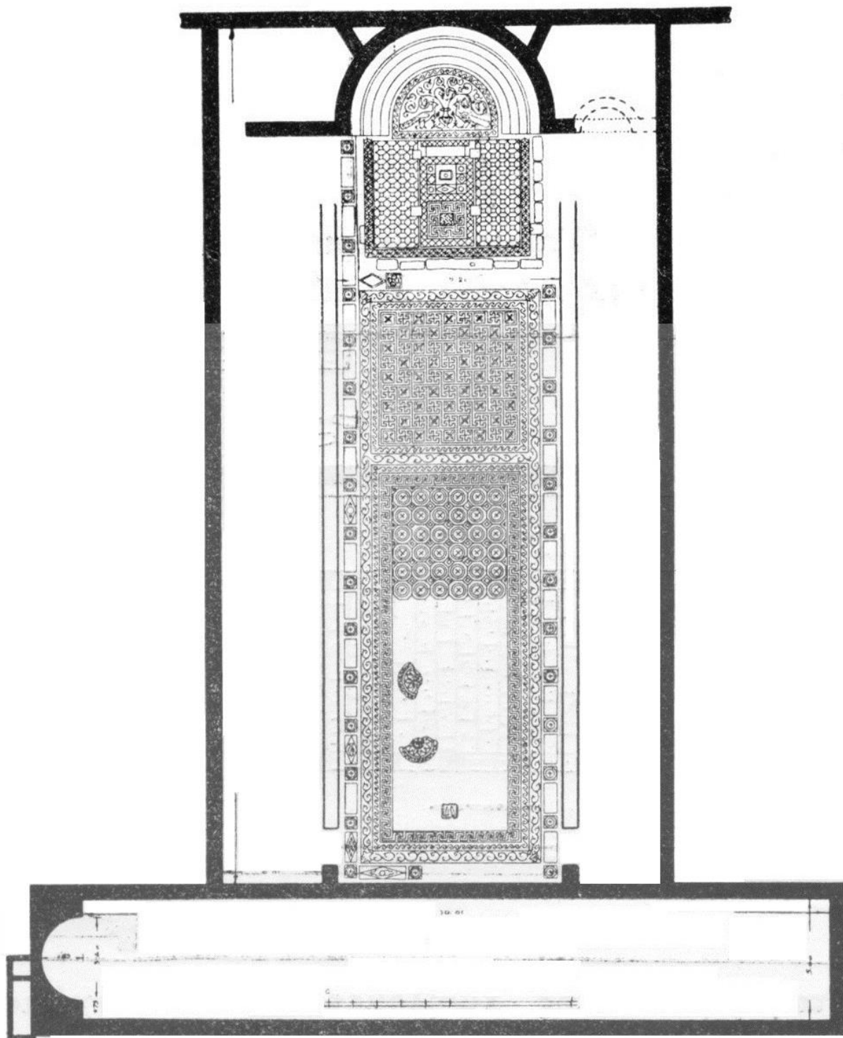
Κάτοψις βασιλικῆς Ἀφεντέλλη κατὰ σχέδιον Ἀν. Ὀρλάνδου. (Εἰκὼν 5).
