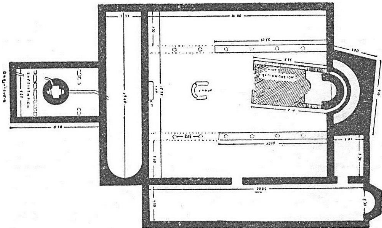
Κάτοψις τῆς βασιλικῆς τῶν Ἀργάλων κατὰ σχέδιον Δ. Εὐαγγελίδη. (Εἰκὼν 6).
