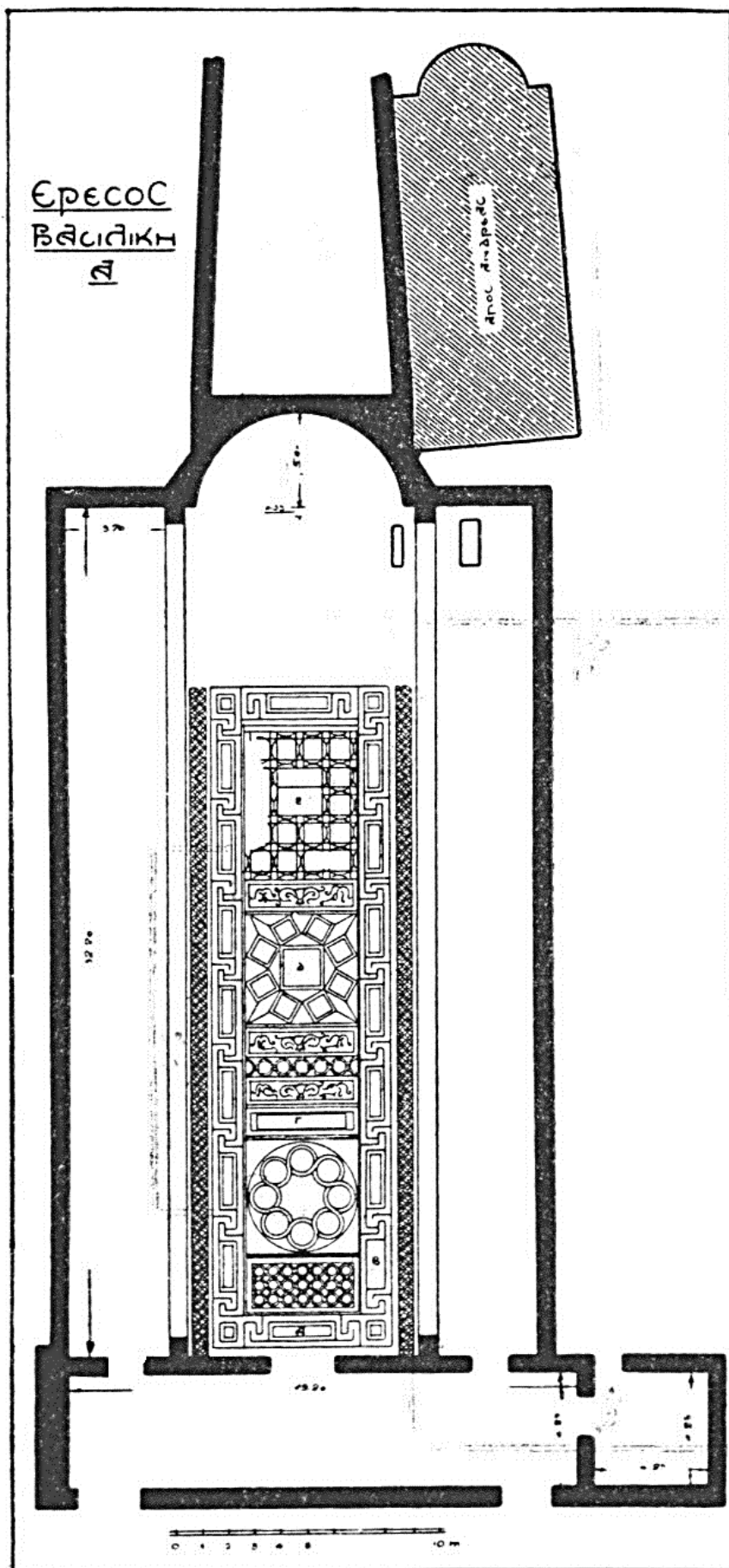
Κάτοψις βασιλικῆς Ἐρεσοῦ κατὰ σχέδιον Ἀν. Ὀρλάνδου. (Εἰκὼν 4).
