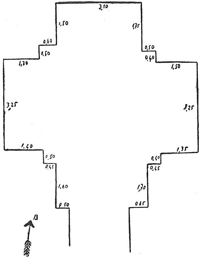
Ὑπόγειος νεκρικός θάλαμος εἰς τὸ Βουναράκι Μυτιλήνης. (Εἰκὼν 2).
