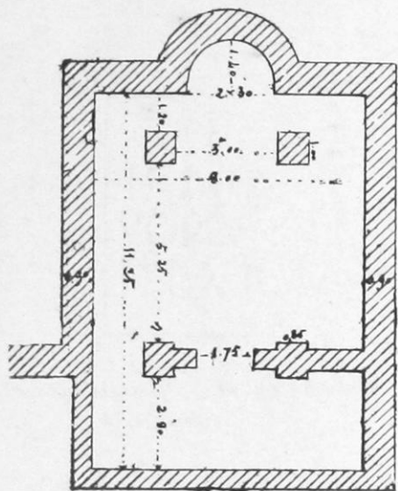
Σχεδιάγραμμα Ἁγίου Χριστοφόρου
