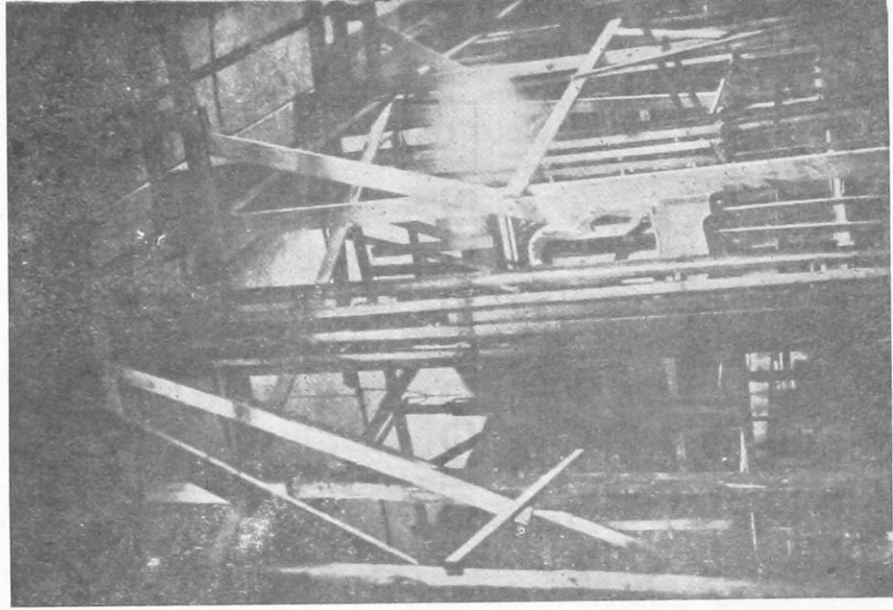
ΑΠΟΨΙΣ ΤΗΣ ΣΤΕΓΗΣ ΚΑΙ ΤΟΥ ΕΣΩΤΕΡΙΚΟΥ ΤΟΥ ΚΥΡΙΩΣ ΝΑΟΥ ΕΠΙΣΚΕΥΑΖΟΜΕΝΟΥ
